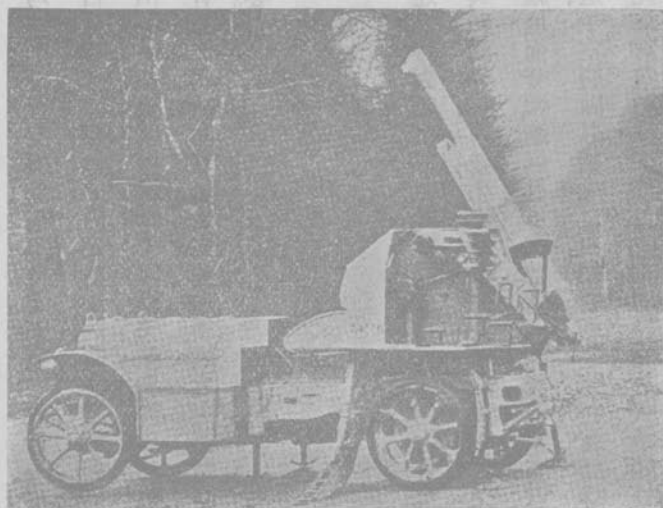
圖三十第 自動高射炮
