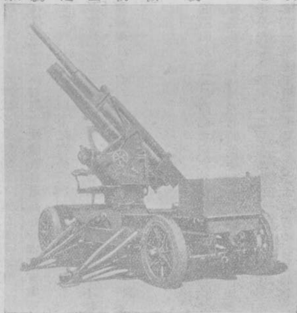
圖二十第 美國式自動高射炮
